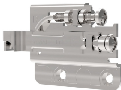
QSS Element de suspendare 704, max 40kg, dreapta
