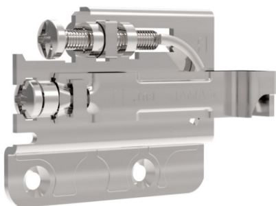
QSS Element de suspendare 704, max 40kg, stânga
