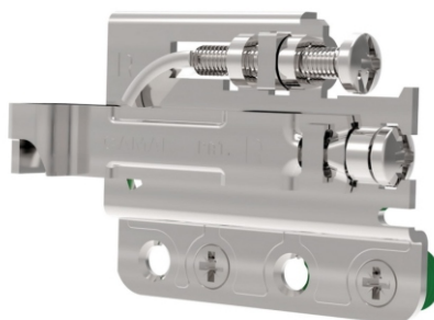
QSS Element de suspendare 704 cu diblu, max 77kg, dreapta
