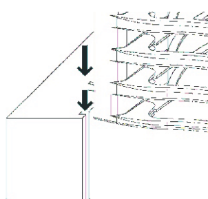
Montare în canal frezat
