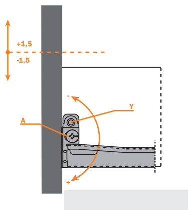
mod de reglare fațetă
