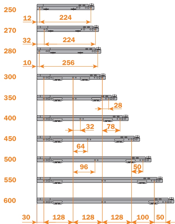
schema de găurire sertar
