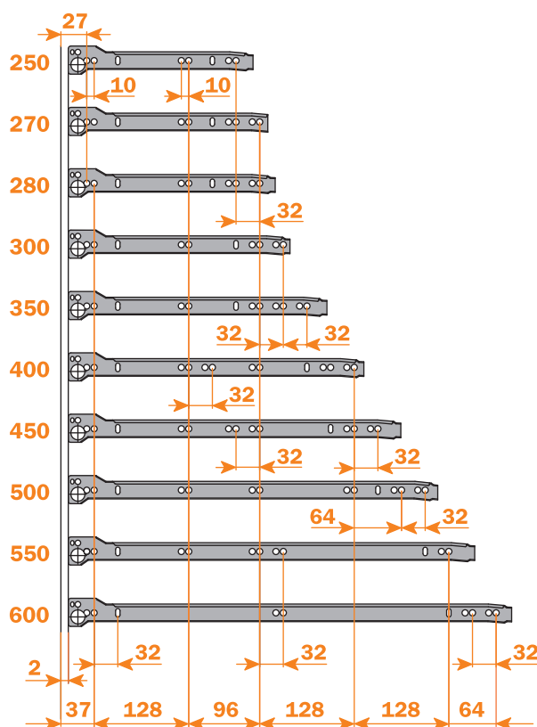
schema de găurire laterală corp
