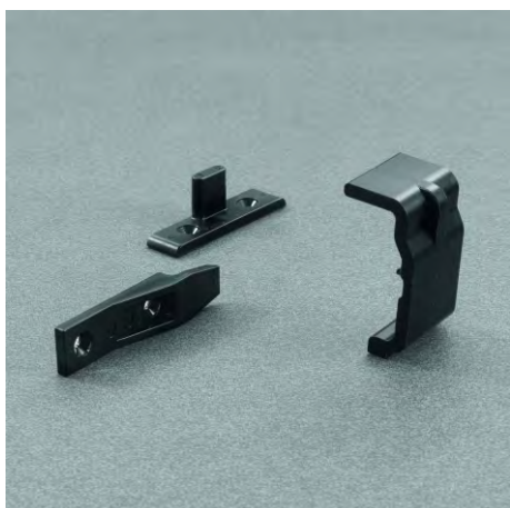
Element de rigidizare pentru fund sertar lat
