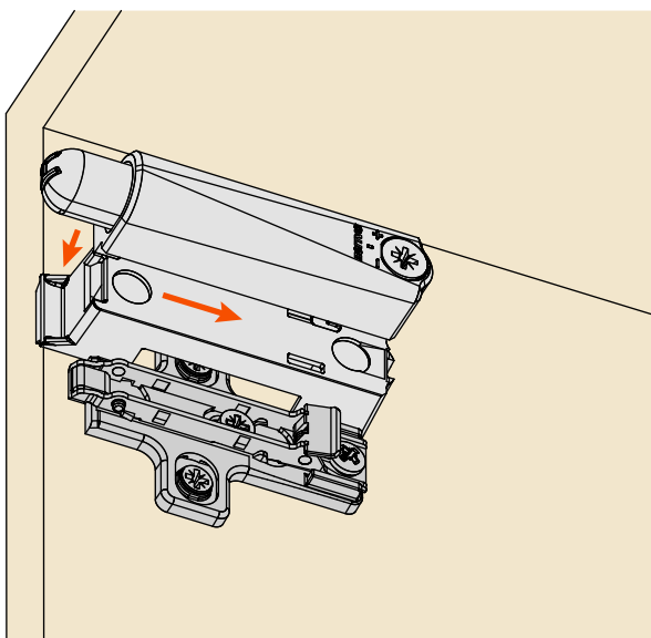
Montarea amortizorului
