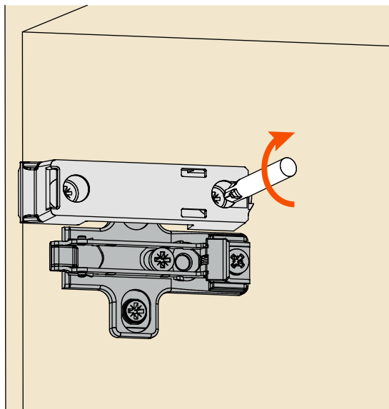
Înșurubarea pe laterală
