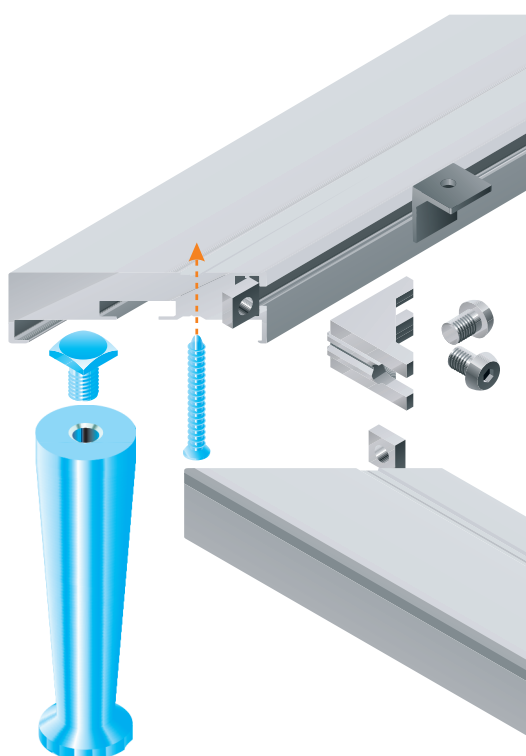
PMO.3005N picior aluminiu cu Ø40mm
