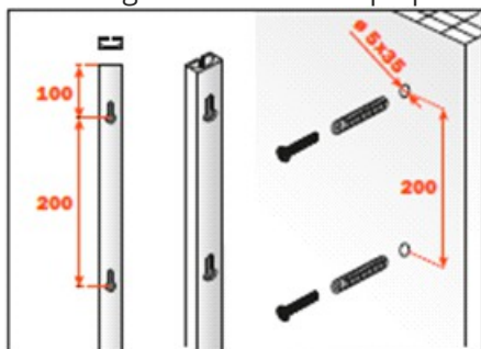
Cote de găurire - montare pe perete
