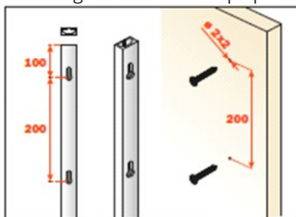
Cote de găurire - montare pe panou
